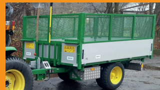
TA 140 / 160 / 190 / 210 - 14 / 16 / 19 / 21 To. 500 / 600 / 650 / 700 / 750 / 820 x 250 / 255 cm mit Bordwänden und Rampen / avec ridelles et rampes
